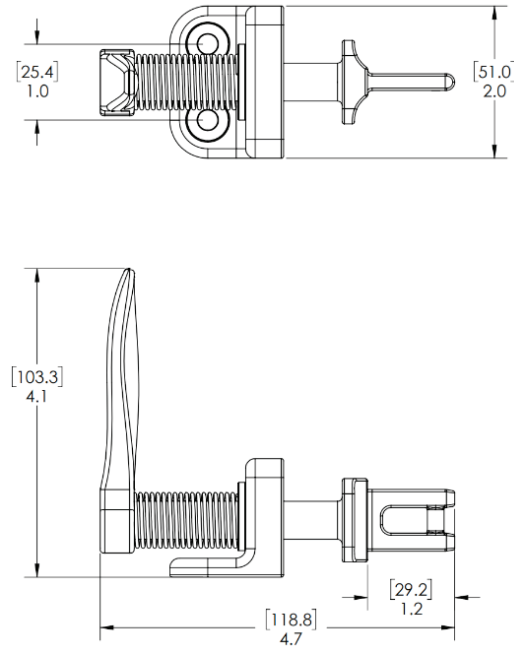
Type DS (Latch)
