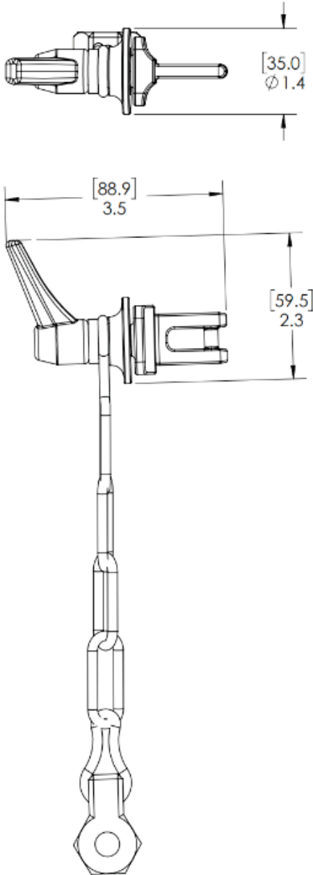
Type DS (Chain Latch)
